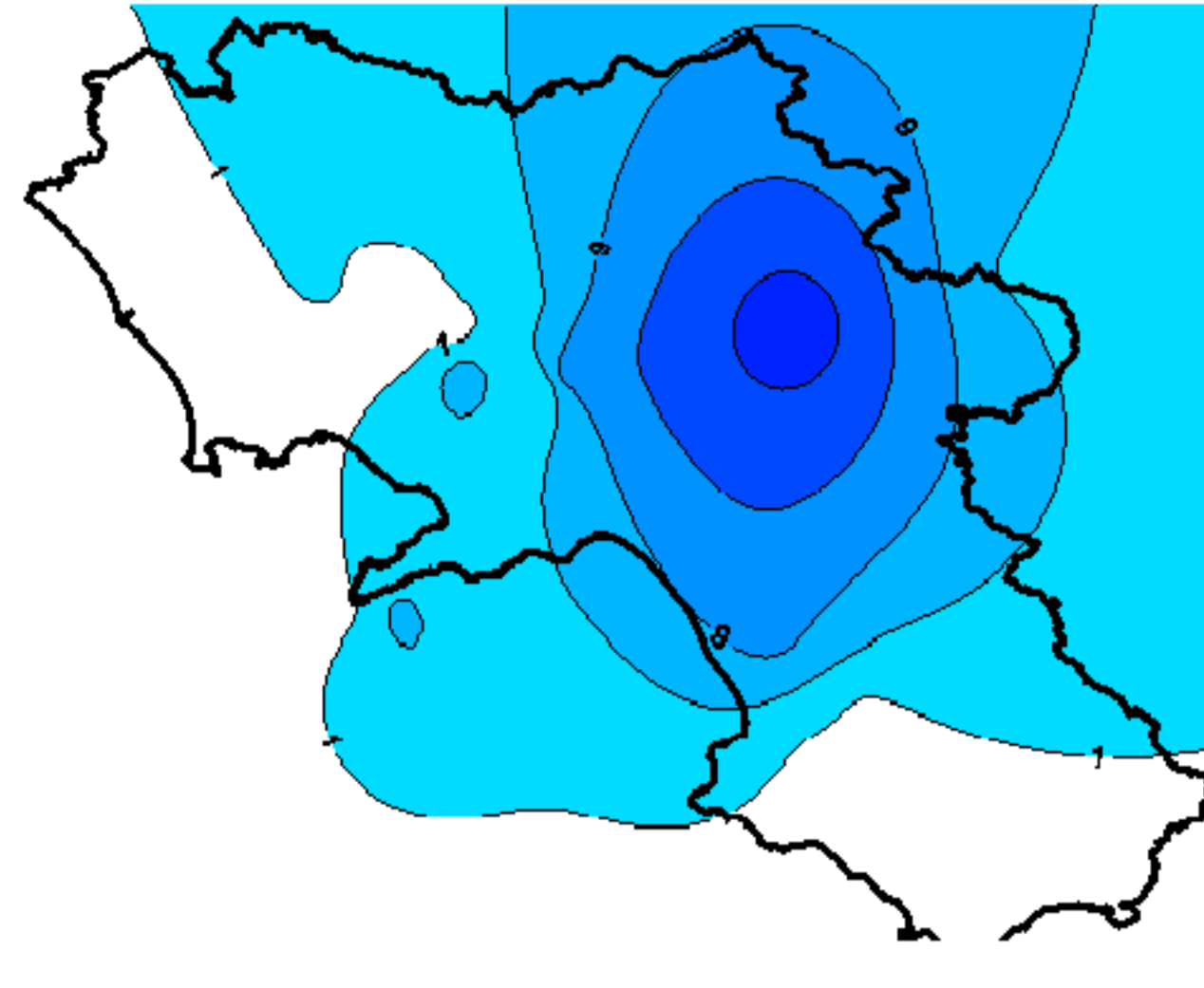
Precipitazioni mm/24h
